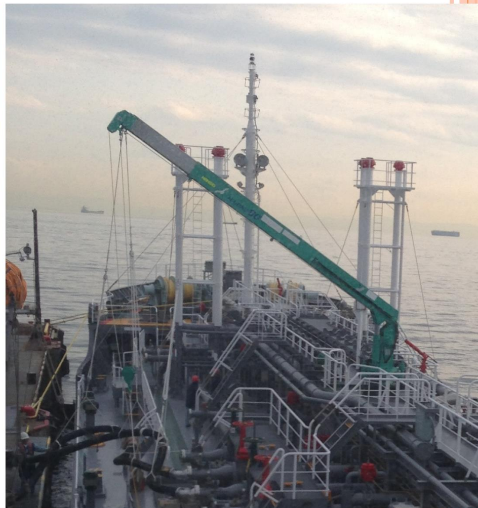
カーゴホースによる荷役 本船のカーゴホース・クレーンによる荷役
